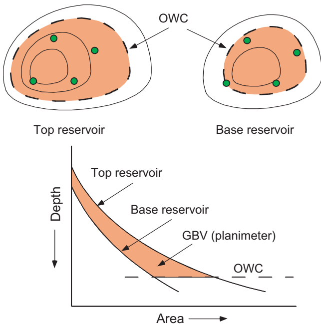
Fig. 7—Estimating GBV.
